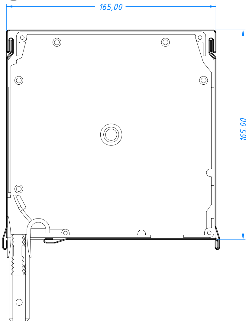
332010 CAJON ALUMINIO PERFILADO 4P 165
